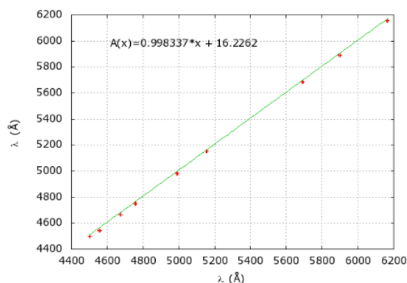
Сурет 1. Эксперимент үшін калибрлеу қисығы
