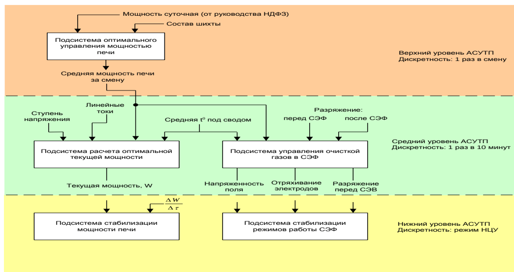
Сурет 1. Сары фосфор өндіру процесін оңтайлы бақылау жүйесінің үш деңгейлі иерархиялық құрылымы
