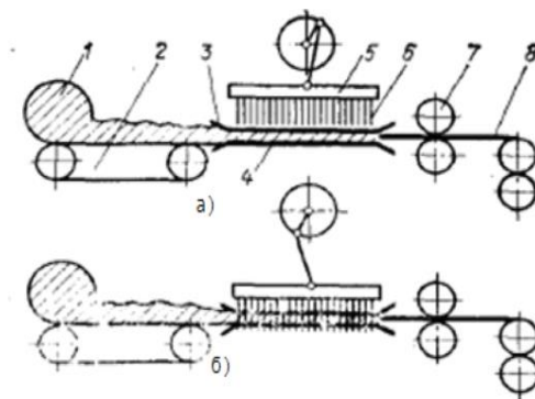
Сурет 5. Ине тесетін машинаның жұмыс схемасы
