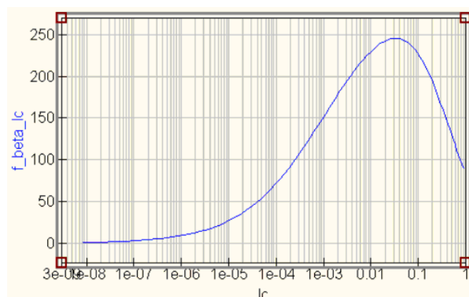
Сурет 4. Транзистордың коллектор тогының шамасынан ток бойынша күшейту коэффициентінің тәуелділік графигі
