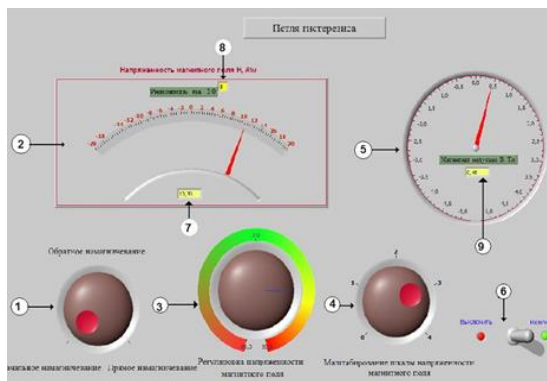
Сурет 2. Гистерезис ілмегін LabView бағдарламасында зерттейтін беттік панель
