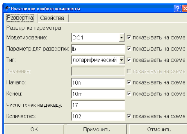
Сурет 2. Параметрді ашу бойынша модельдеу қасиеттерінің көрінісі
