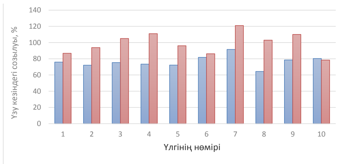
Сурет 3. Беймата материалдарды ұзу кезіндегі ұзару, %
