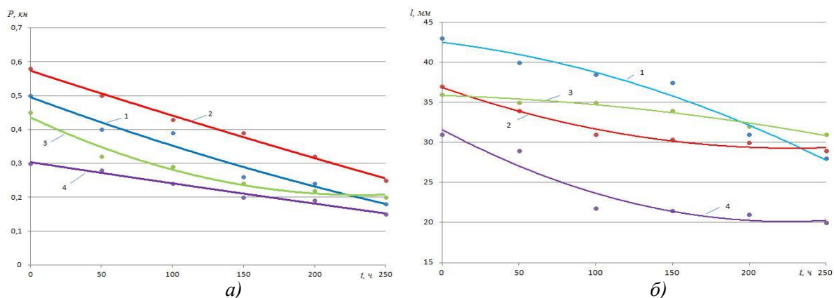
Сурет 1. Судың жіпті тігістің үзілу кезіне әсер ету уақыты (а) және тігістің үзілу кезіндегі ұзаруына әсері (б): 1 – қаймалы бастырма тігіс, 2- қайма тігіс, 3 – бастырма тігіс, 4 – айкаспа тігіс
