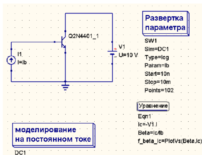
Сурет 1. Параметрлері ашылған модельдеуді орындау үшін сызықты емес элементі бар тізбек
