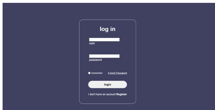
Рисунок 1. Авторизация пользователя
