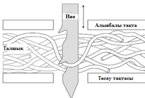
Сурет 4. Тескіш иненің әрекеті
