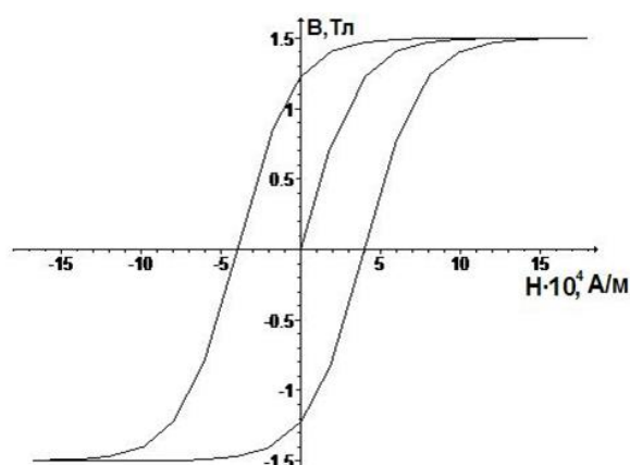
Сурет 4. Гистерезис ілмегінің графигі
