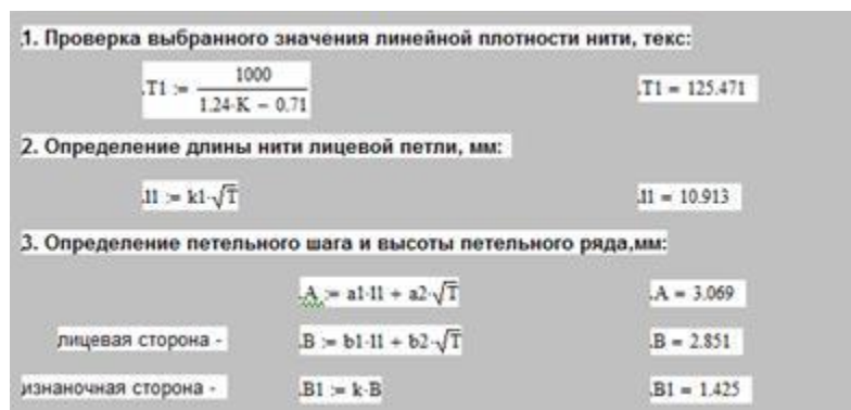
Сурет 2. Mathcad есептеуіш ортасында jacquard тоқыма контурының параметрлерін есептеу
