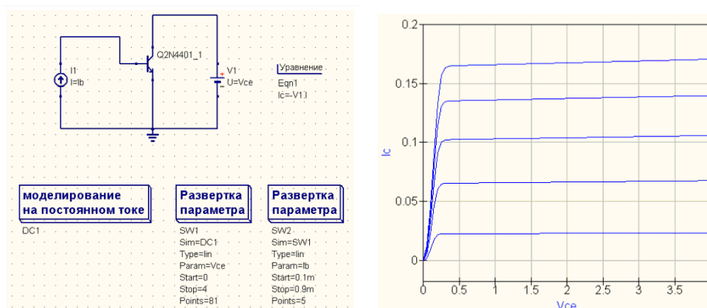
Сурет 5. Биполярлы транзистордың шығыстық сипаттамасының принципиалды схемасы (а) және вольтамперлік сипаттамасының диаграммасы (б)
