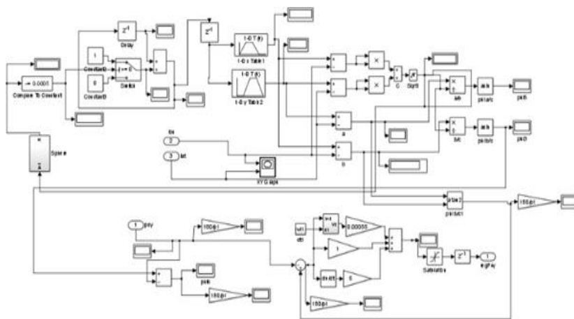
Рисунок 3. Схема автопилота в Matlab Simulink
