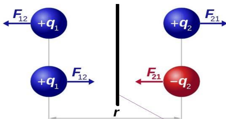
Сурет 1. Электр өрісіндегі кулон күші
