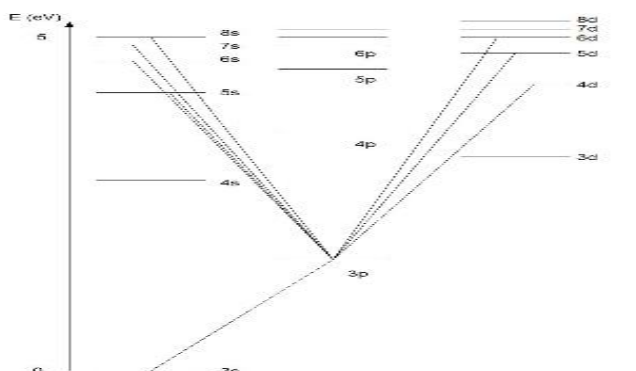
Сурет 2. Натрийдің көрінетін спектрінің готтриандық диаграммасы
